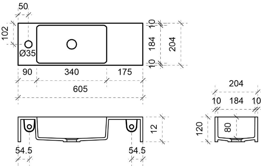
TEKENING 1200
