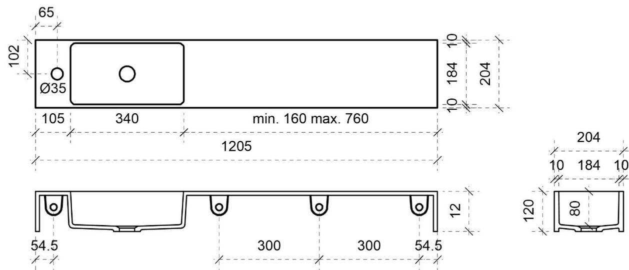
TEKENING 1200
